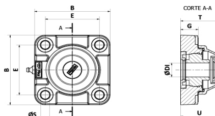
Caja porta rodamiento - 4 agujeros - Negro (UCF) - Rodamiento (UC) / (S-UC) Inoxidable.
