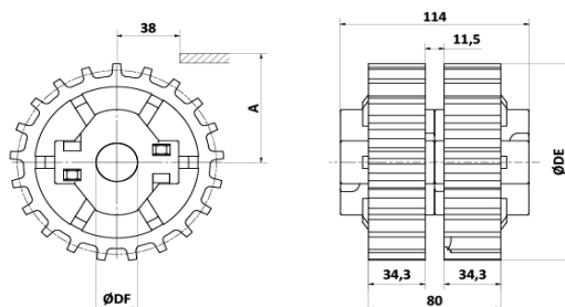
Piñón Asimétrico Serie 821 - Sin chavetero
